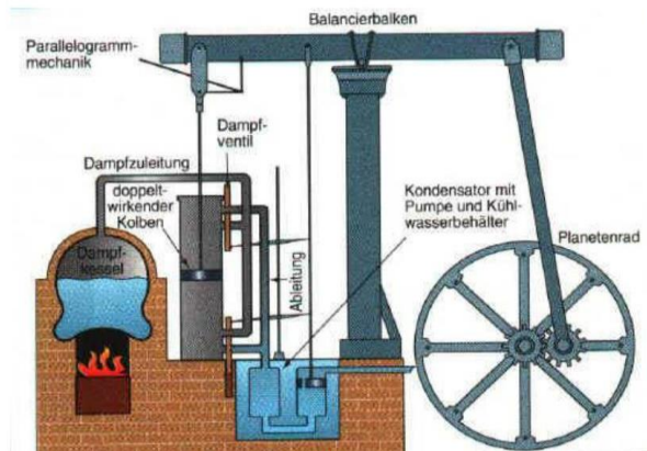
Die Dampfmaschine nach Watt (1776/1782)
